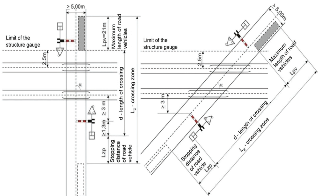
Slika 1. Prelaz u nivou sa uglom ukrštanja: a = 90^\circ (levo) i a < 90^\circ (desno) [6,7].
